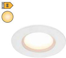
Dorado 1-Kit 49430101 White | Metal LED Module 4,7W | 345lm | 2700K H: 3,6 cm | Ø: 8,5 cm
