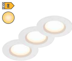
Dorado 3-Kit 49410101 White | Metal LED Module 4,7W | 345lm | 2700K H: 3,6 cm | Ø: 8,5 cm
